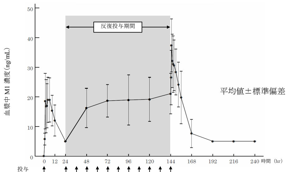
1 回 50mg 投与 血漿中 M1 濃度
